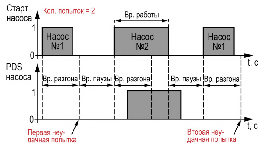
Рисунок 13.9 – Перезапуск насоса
