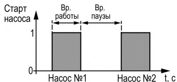
Рисунок 13.8 – Чередование насосов
