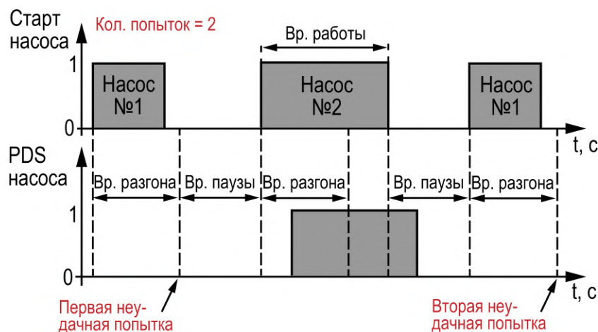
Рисунок 14.8 – Перезапуск насоса
