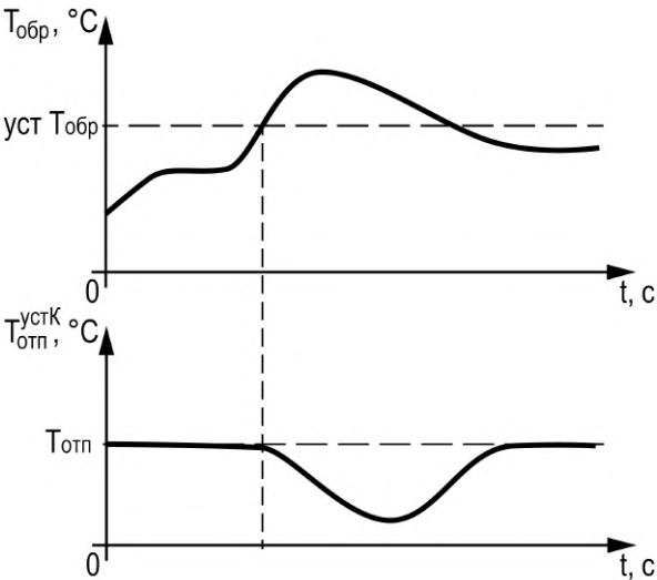
Рисунок 13.4 – Коррекция температуры отопления
