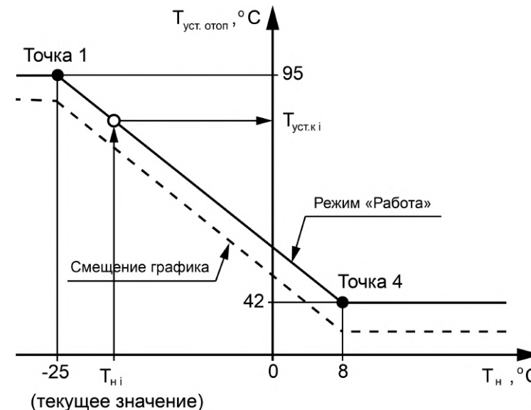
Рисунок 13.3 – Отопительный график
