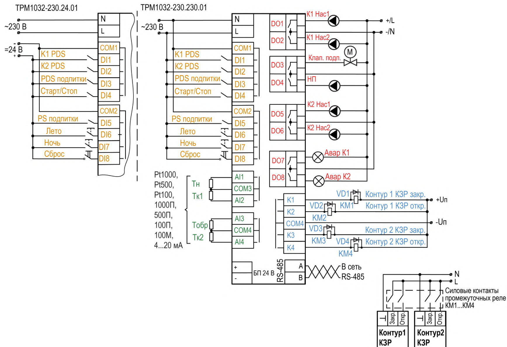
Рисунок 9.3 – Схема подключения
